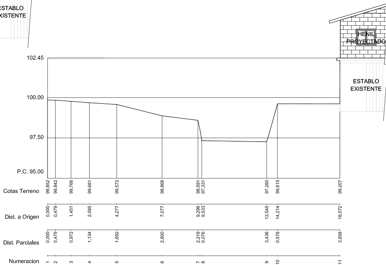
PERFIL 2
