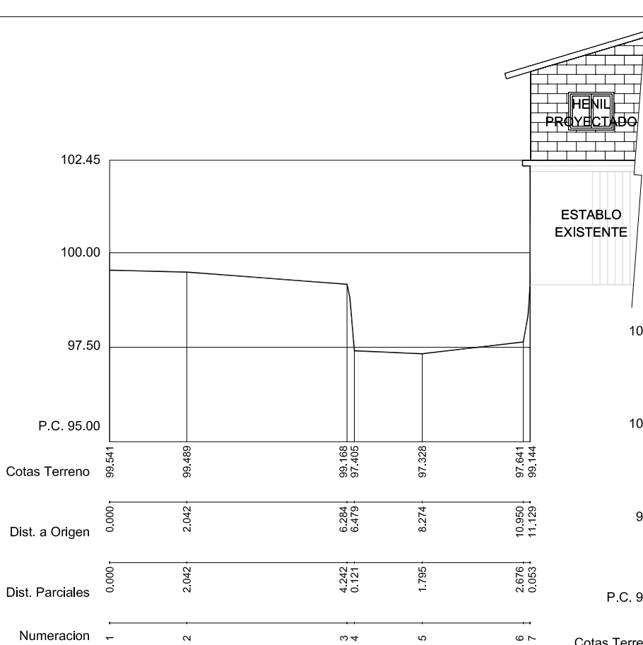
PERFIL 1
