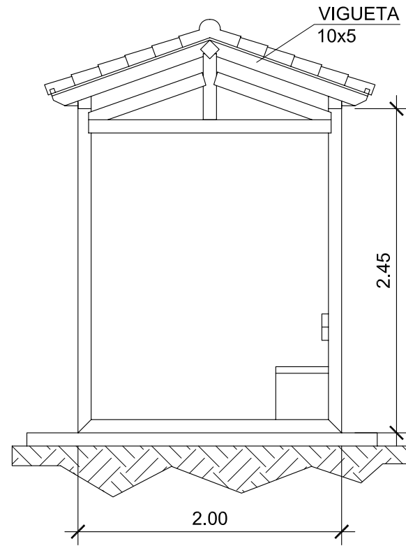
VISTA LATERAL
