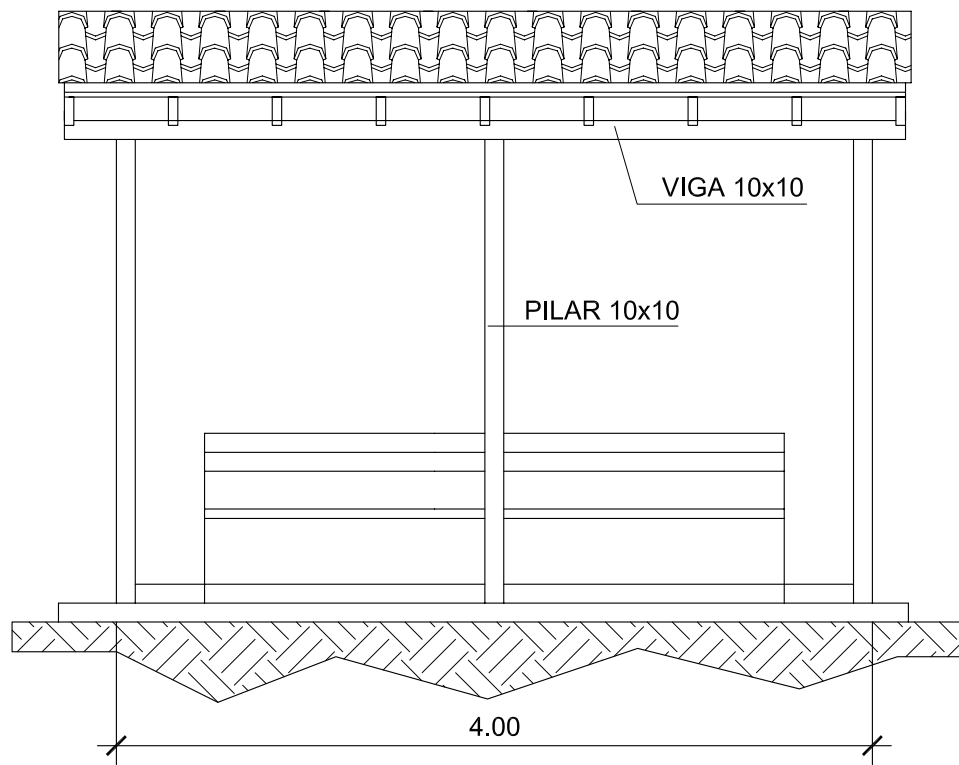
ALZADO
